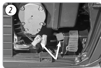
2. Під'єднайте мінус акумулятора шляхом з'єднання його кабелю.
